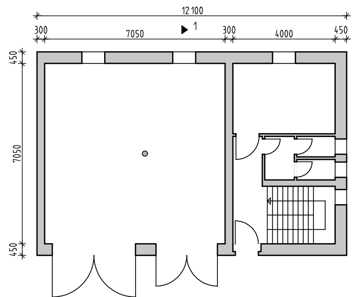
1.NP
