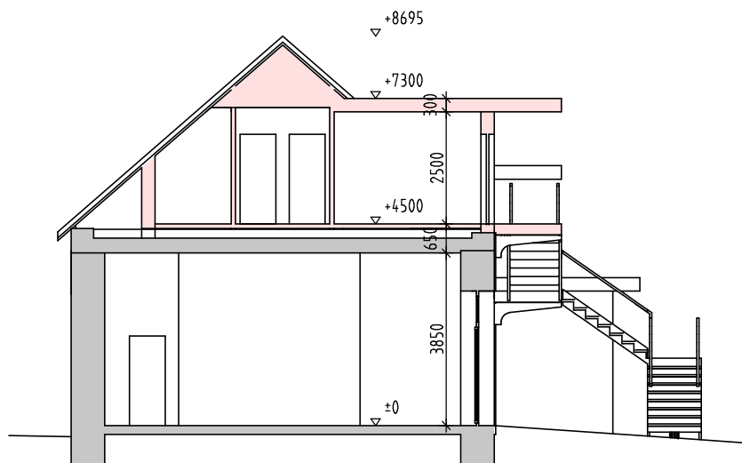
ŘEZ 2
