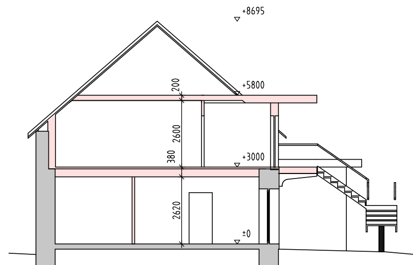
ŘEZ 3
