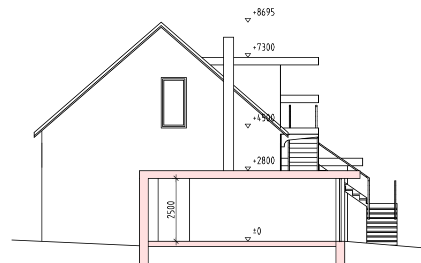
ŘEZ 1
