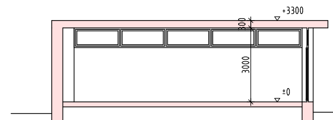
ŘEZ 4
